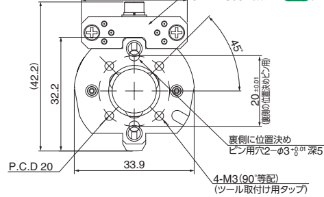
140329 OX-005用接続コネクター(ツール側) OXR-PS06-1(別売品(1-31))
