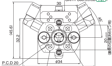
4-φ3.2, φ6.5ザグリ深3.3(90°等配) (ロボット取付け穴)
