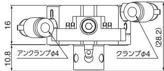
140328 OX-005用コネクター(ロボット側) OXR-PS06(別売品(1-31))
