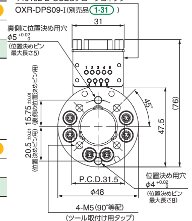
140192 D-SUB&プローブコネクター OXR-DPS09-1(別売品(1-31))
