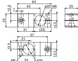
クロスコネクター・ φ20 φ20 (後入)
