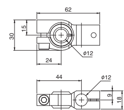
ティーコネクター #1・ φ8 φ12
