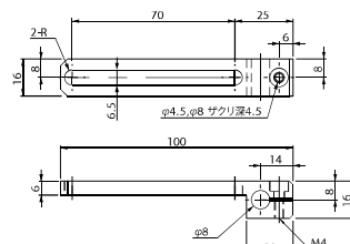
スライド70 ブラケット・ T・φ20
