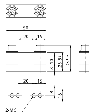
角スライドブラケット・25-25
