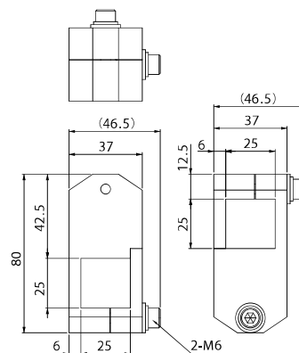
角スライドブラケット・10-20
