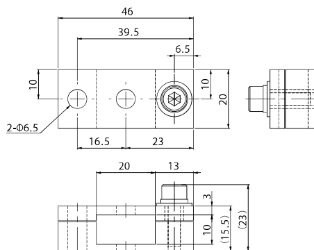
角スライドブラケット・20-10
