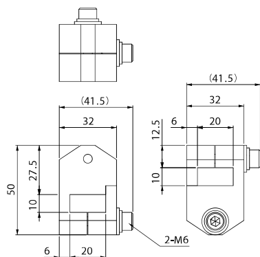
アタッチブラケット・10-20・M6
